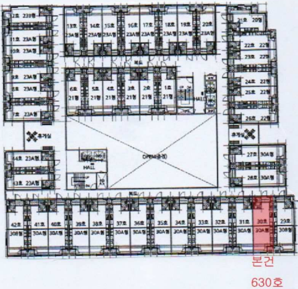
<630호 내부구조도>
