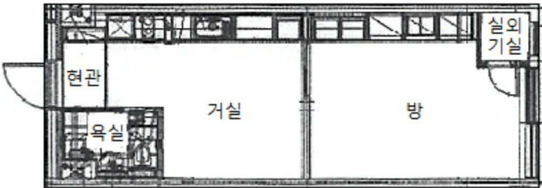
<내부구조도>
