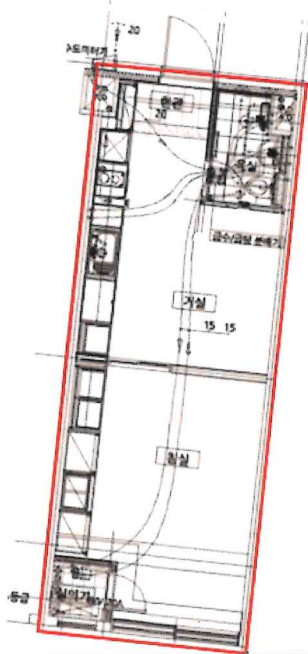
< 제539호 내부구조도 >
