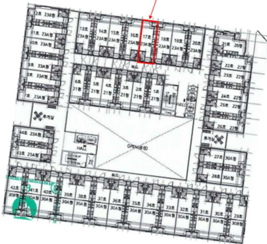
<호별배치도>
