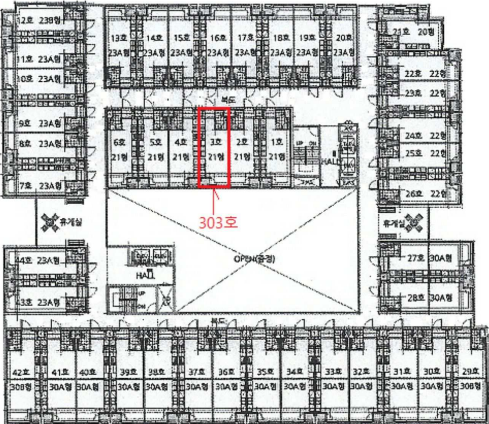
<호별배치도>
