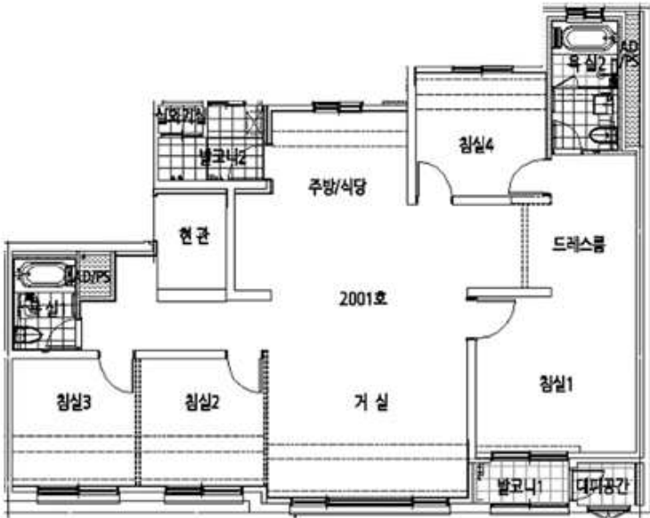
【 2001호 내부구조도 】
