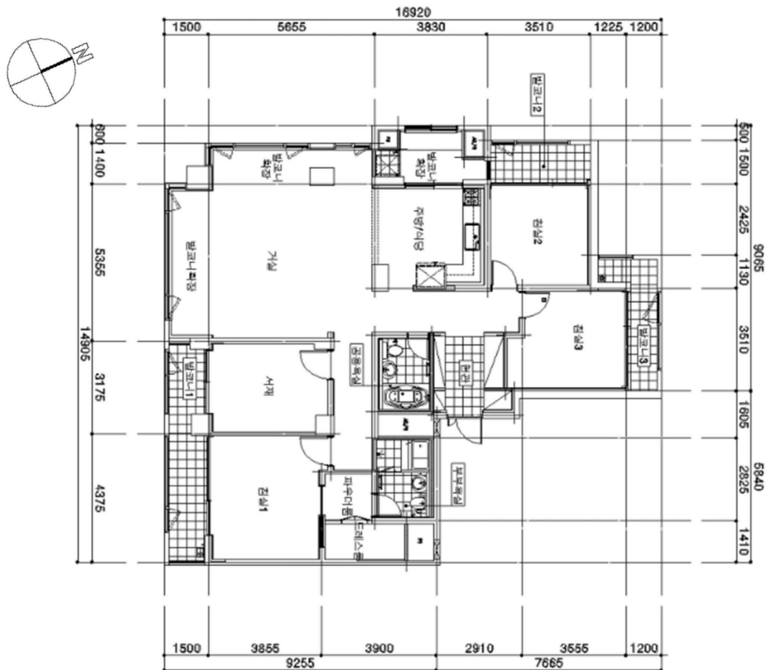
<제103호 내부구조도>
