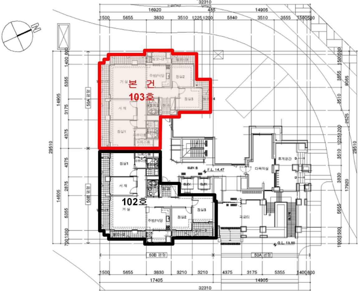
<제1층 호별배치도>
